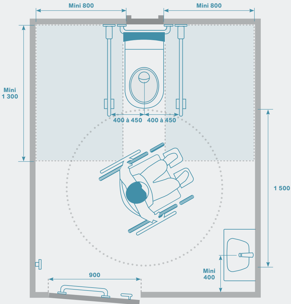
Installation alternative permettant le transfert à droite et à gauche
