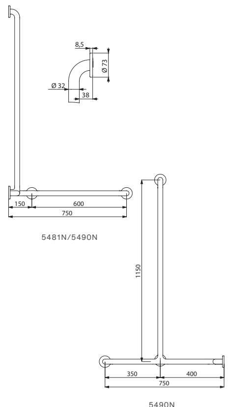
Emplacement de la remontée réglable à gauche ou à droite (réf. 5481N)
