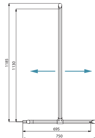
Emplacement de la remontée réglable à gauche ou à droite
