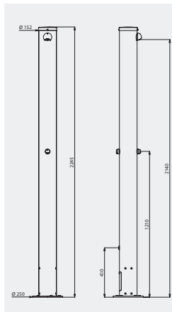
Colonne de douche PLEIN AIR avec 1 douche et 1 rince pieds Réf. DELABIE : 717511
