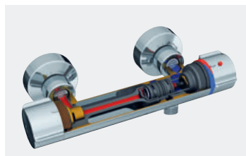
Coupe H9769 : faible volume d'eau, isolation thermique et absence de clapet antiretour Réf. DELABIE : Coupe3D_H9769
